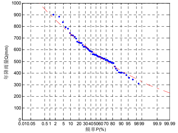
图2 西安1951-2003年降雨量P-III频率曲线。
